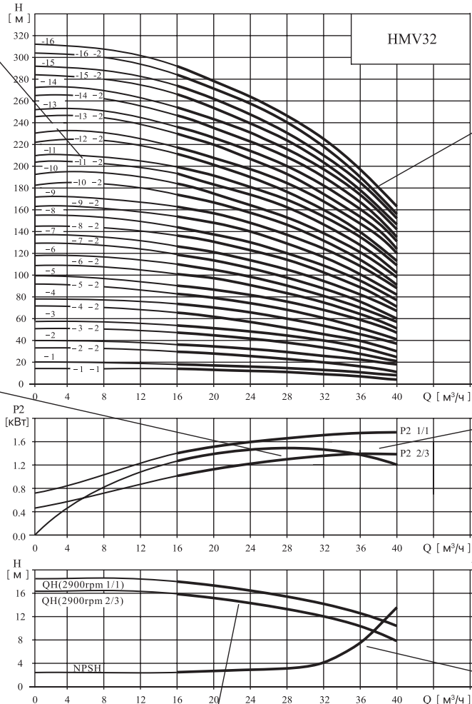
График характеристики «Q-N» для каждого отдельного рабочего колеса. Представлены графики для рабочих колес стандартного (1/1) и уменьшенного (2/3) диаметров.
